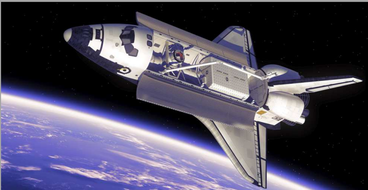
lo shuttle
