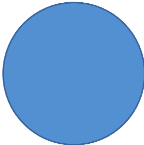
circle
